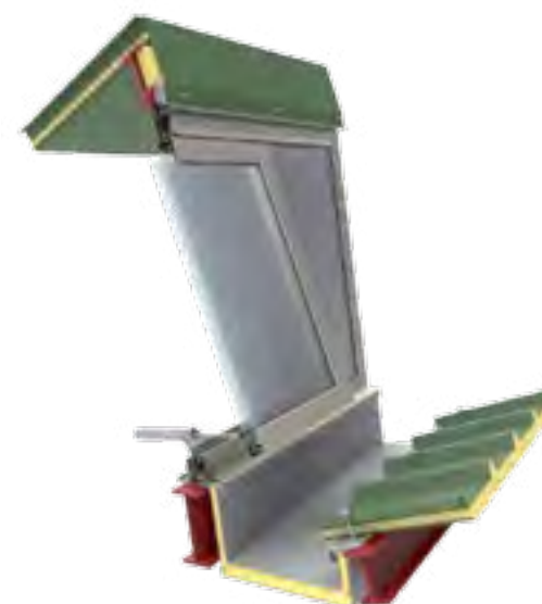
PROFILE CU BARIERĂ TERMICĂ Utilizarea noilor profile cu barieră termică garantează o etanșare perfectă împotriva agenților atmosferici prin evitarea disipării căldurii.
